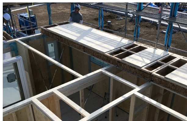
墜落・転落災害防止のために、2階床に合板付きの床パネルを採用（写真3）。
